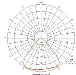
Curva fotométrica
